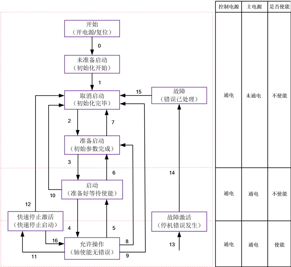
图 7.1 CL3B 的 402 状态机
