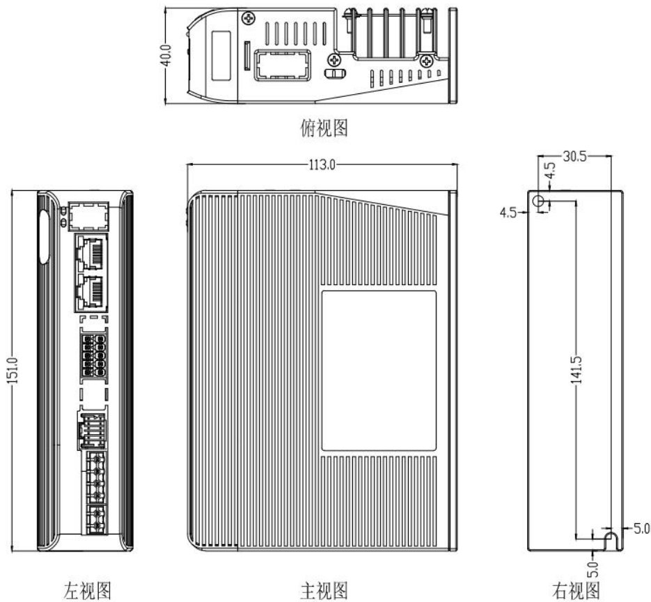
图 2-1 CL3B-EC808AC 安装尺寸图(单位：mm) ※ 设计安装尺寸时，注意考虑端子大小及布线！
