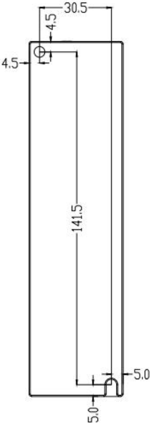
图 2-1 CL3B-EC808AC 安装尺寸图(单位：mm) ※ 设计安装尺寸时，注意考虑端子大小及布线！
